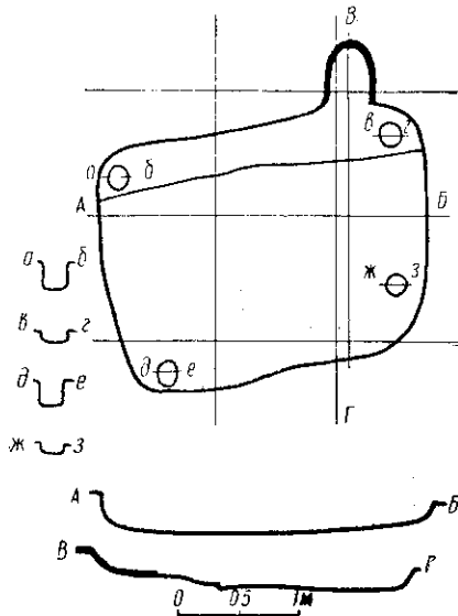
Рис. 1. План і розріз житла № 1.
